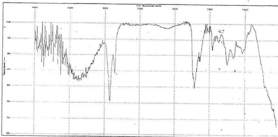
Рис. 1. ИК-спектр поглощения ( 4000-550\text{см}^{-1} ) частиц вещества.
